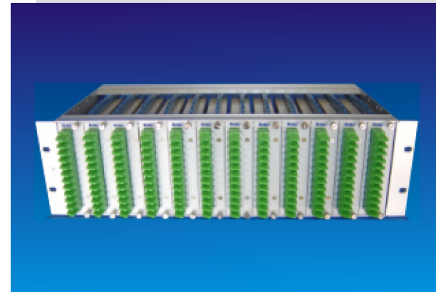
SUB-BASTIDOR EQUIPADO PARA 144 FIBRAS
